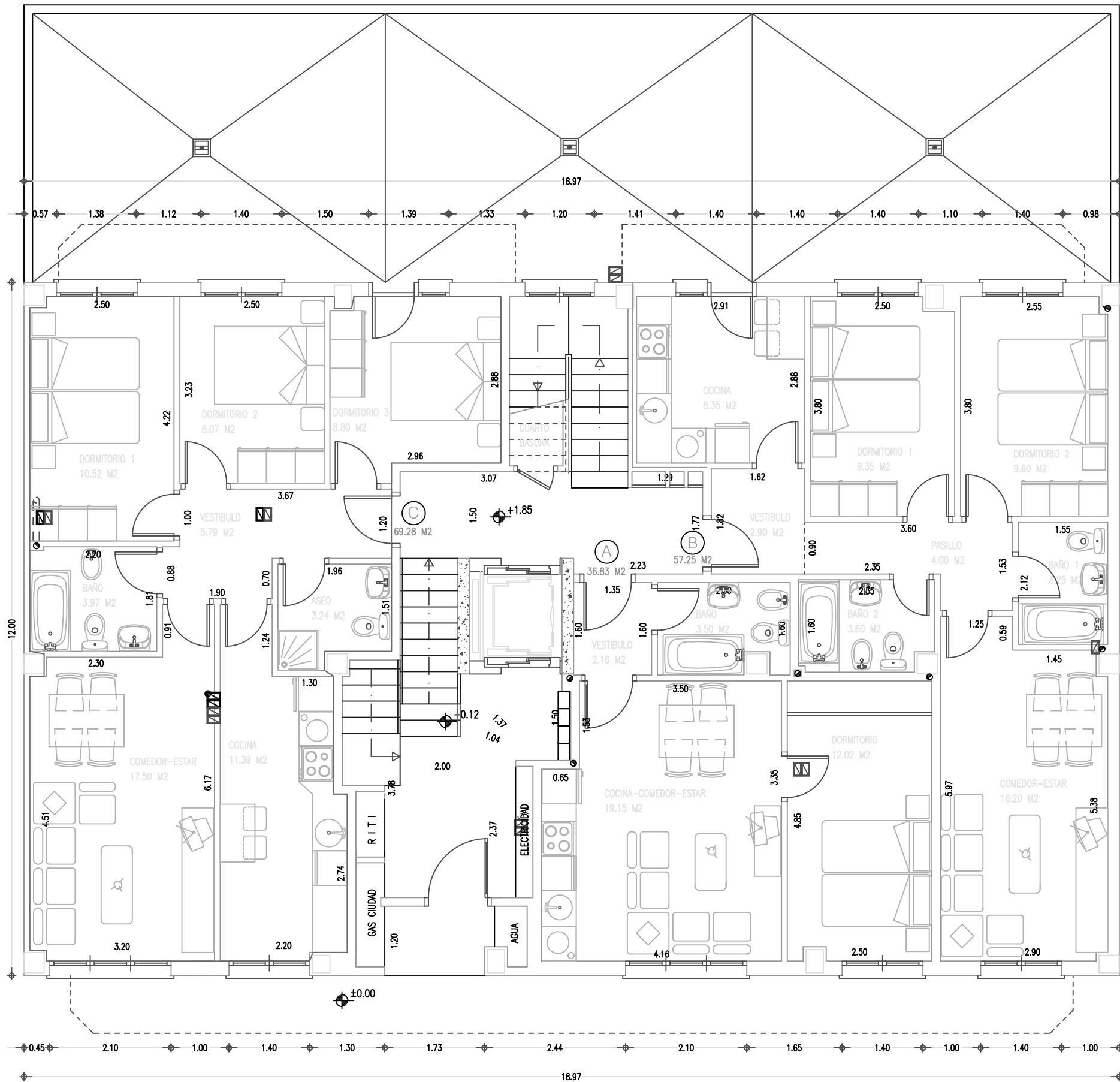
PLANTA BAJA. REPLANTEO DE ALBAÑILERIA Y MOBILIARIO
